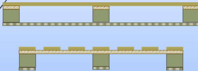
Fig. 3.16 Pallet doble faz con piso inferior sobre patines y tacos
