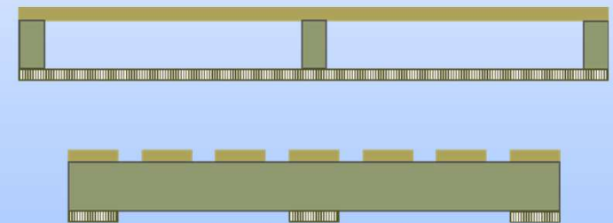
Fig. 3.16 Pallet doble faz con piso inferior sobre patines y tirantes
